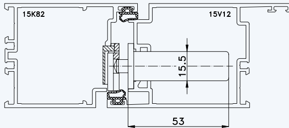
Situation Türfänger (bei Verriegelung mit Türwächter)
