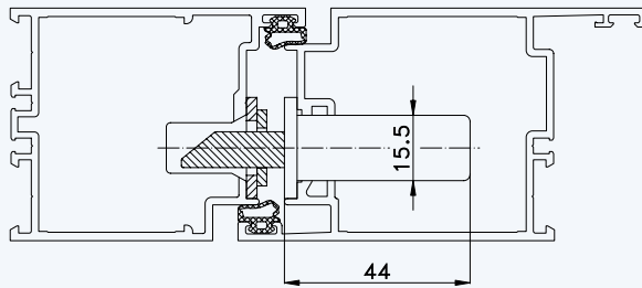
Situation Massivschwenkriegel (bei Automatik-Verriegelung)
