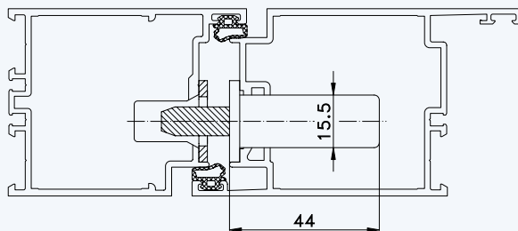
Situation Bolzen (bei Tresor-Bolzen-Verriegelung)
