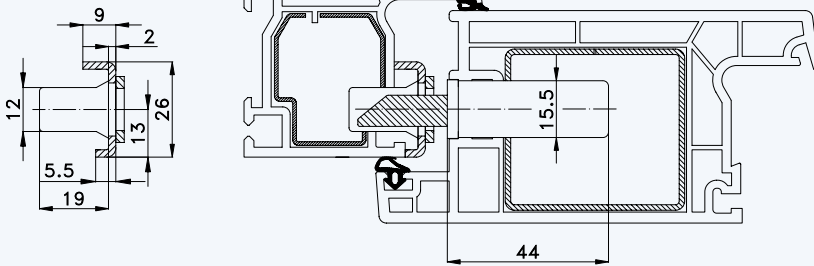
Situation Massivschwenkriegel (bei Automatik-Verriegelung)
