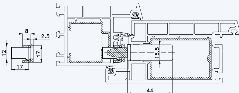
Situation Bolzen (bei Bolzen-Verriegelung)
