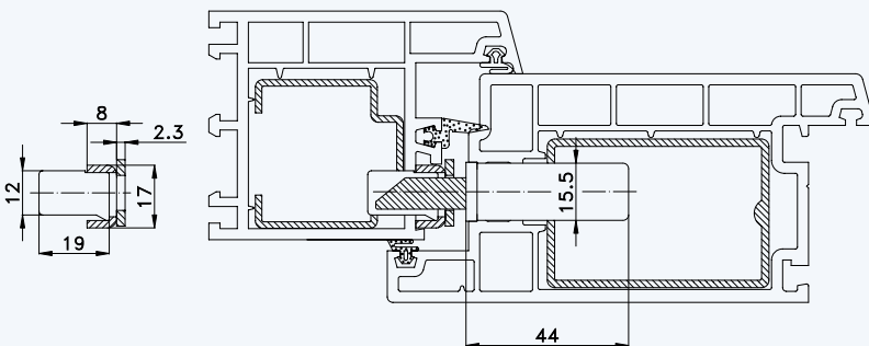
Situation Massivschwenkriegel (bei Automatik-Verriegelung)
