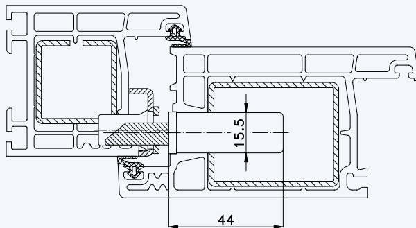
Situation Massivschwenkriegel (bei Automatik-Verriegelung)
