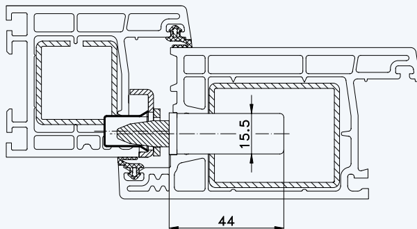
Situation Bolzen (bei Bolzen-Verriegelung)
