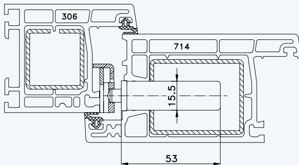
Situation Türfänger (bei Verriegelung mit Türwächter)
