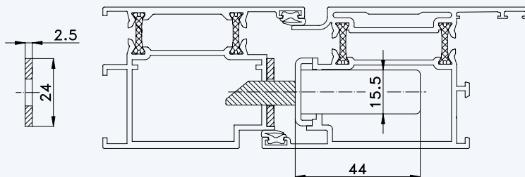
Situation Massivschwenkriegel (bei Automatik-Verriegelung)
