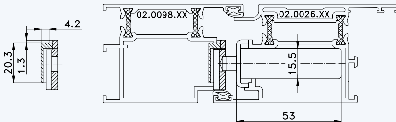
Situation Türfänger (bei Verriegelung mit Türwächter)
