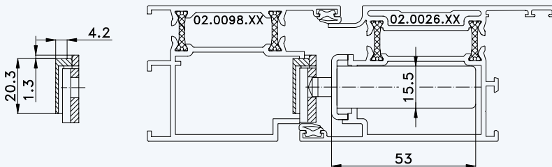
Situation Türfänger (bei Verriegelung mit Türwächter)
