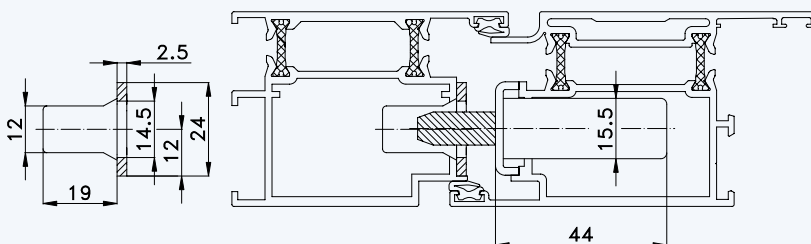
Situation Bolzen (bei Tresor-Bolzen-Verriegelung)
