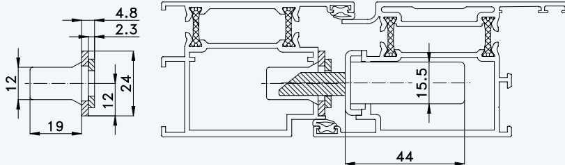
Situation Massivschwenkriegel (bei Automatik-Verriegelung)
