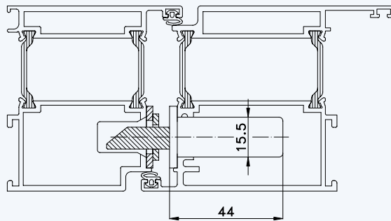
Situation Massivschwenkriegel (bei Automatik-Verriegelung)
