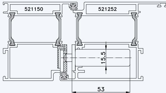
Situation Türfänger (bei Verriegelung mit Türwächter)
