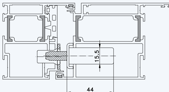
Situation Bolzen (bei Tresor-Bolzen-Verriegelung)
