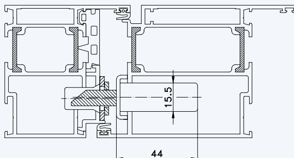
Situation Massivschwenkriegel (bei Automatik-Verriegelung)
