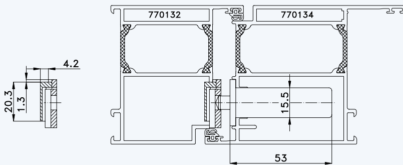
Situation Türfänger (bei Verriegelung mit Türwächter)
