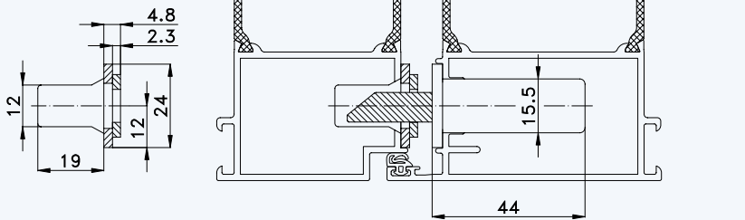
Situation Massivschwenkriegel (bei Automatik-Verriegelung)
